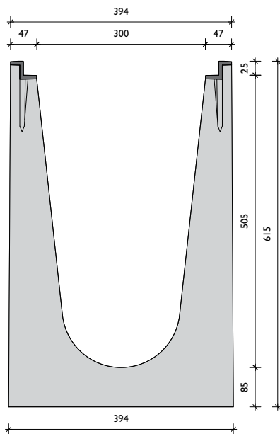
Öntöttvas hosszbordás rács, Oszt. E
