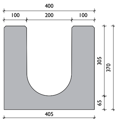
BG Egyedi folyóka NM 200
