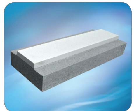
BG-TK Tűzálló fedlap (csak TK1-nél) (A fedlap a jobb láthatóság miatt fejjel lefelé látható)
